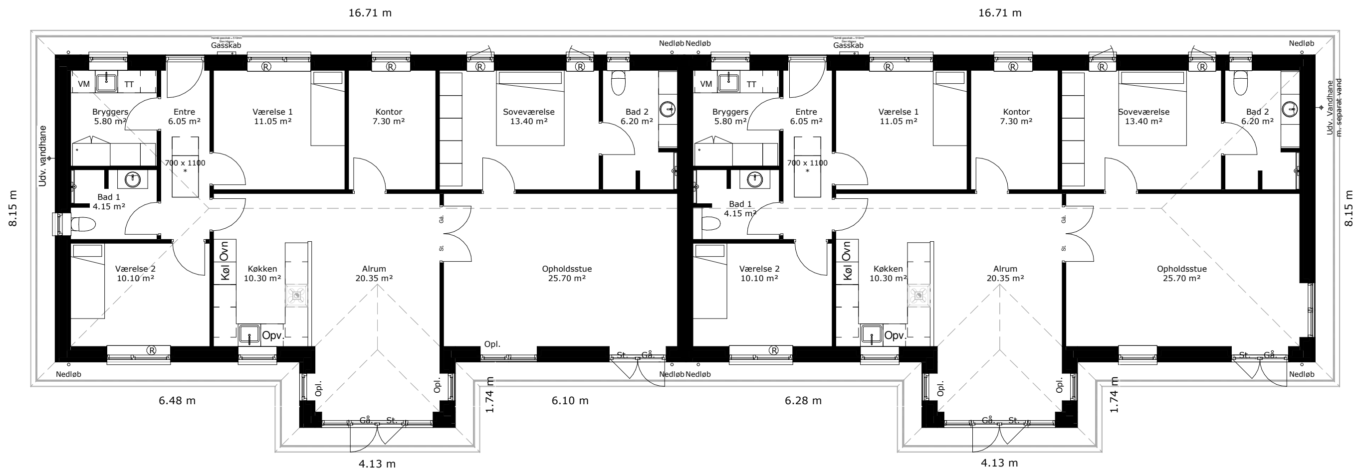
B - Skitse_Stueplan 1 : 100
